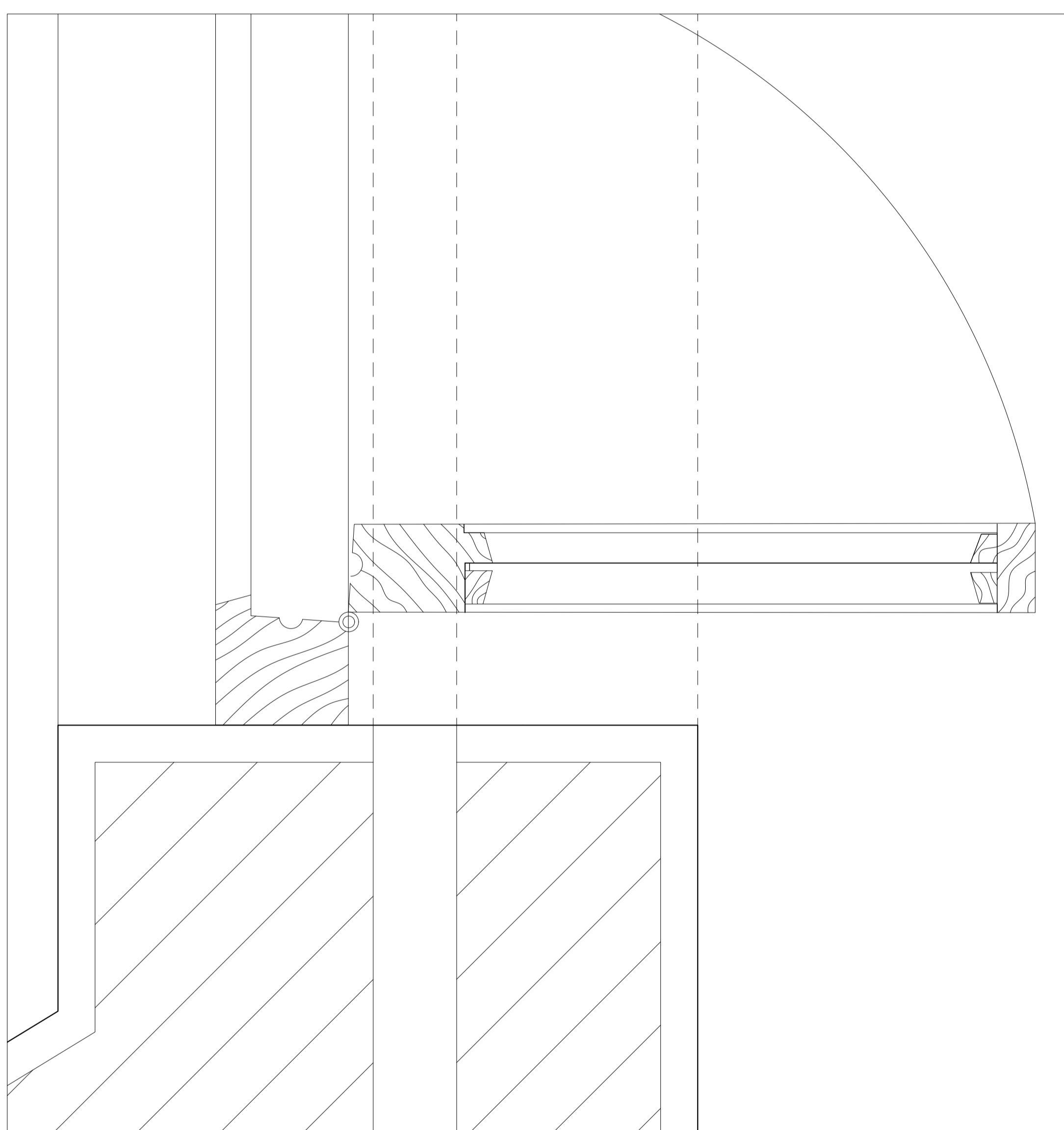
Detalhe de caixilhos de madeira 1:2
