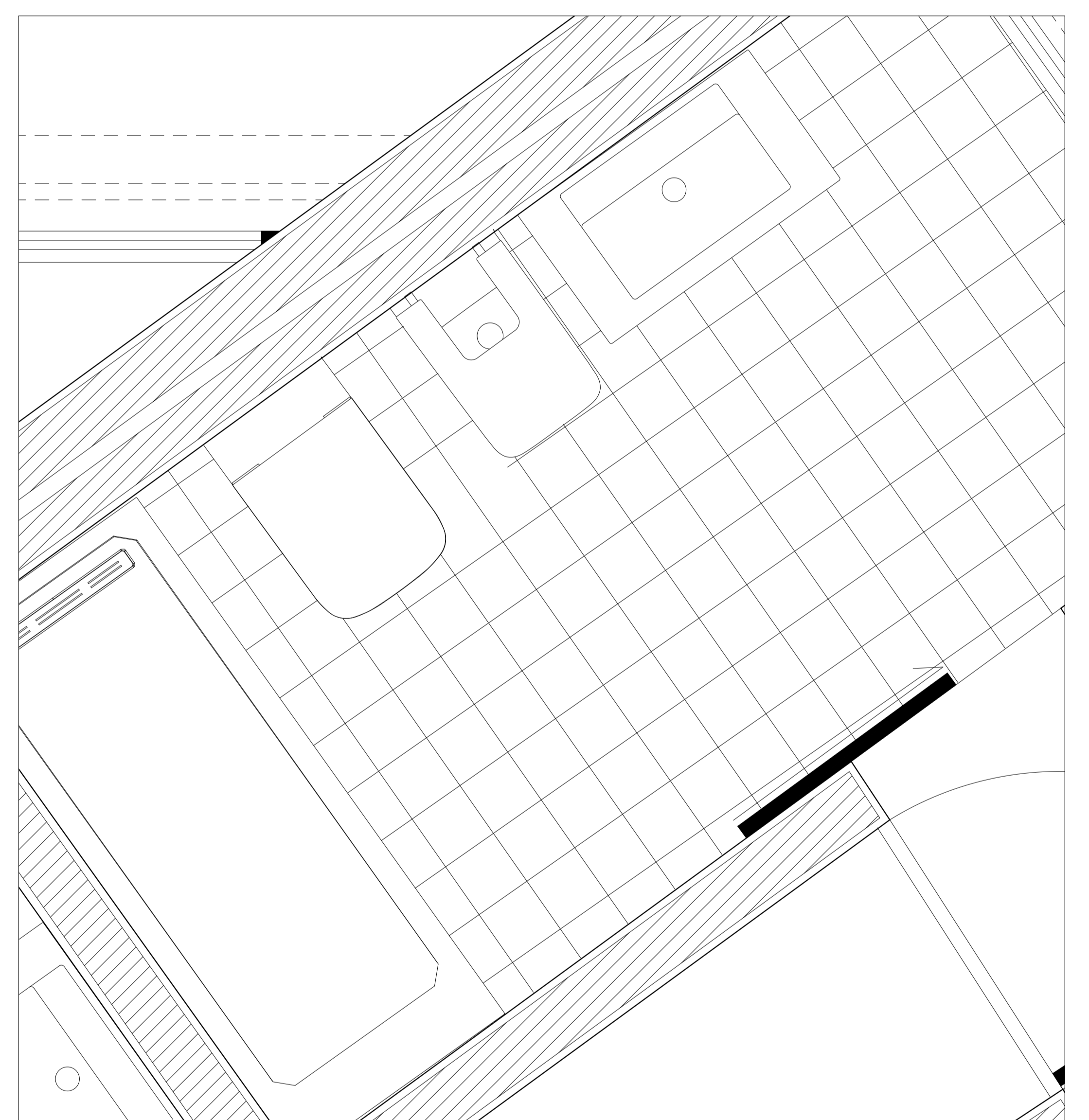
Detalhe da casa de banho 1:10
