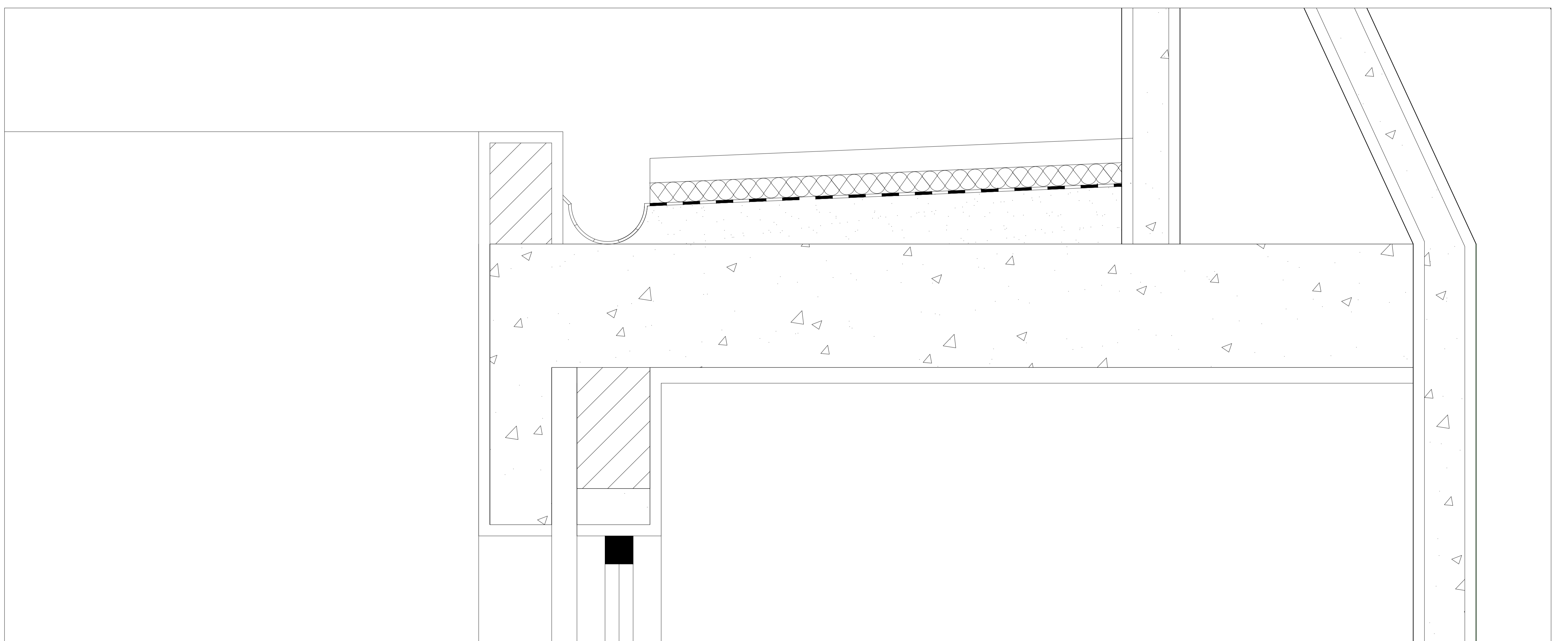
Detalhe da cobertura 1:4
